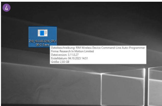
4 exe.-Datei ausführen.
